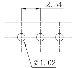
P. C. B. Hole Layout
