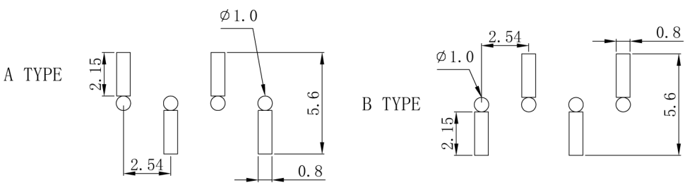
P. C. B. Hole Layout
