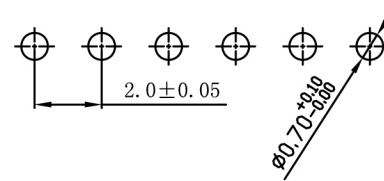
P. C. B. Hole Layout
