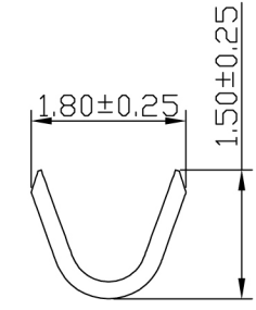
SEC: A-A
